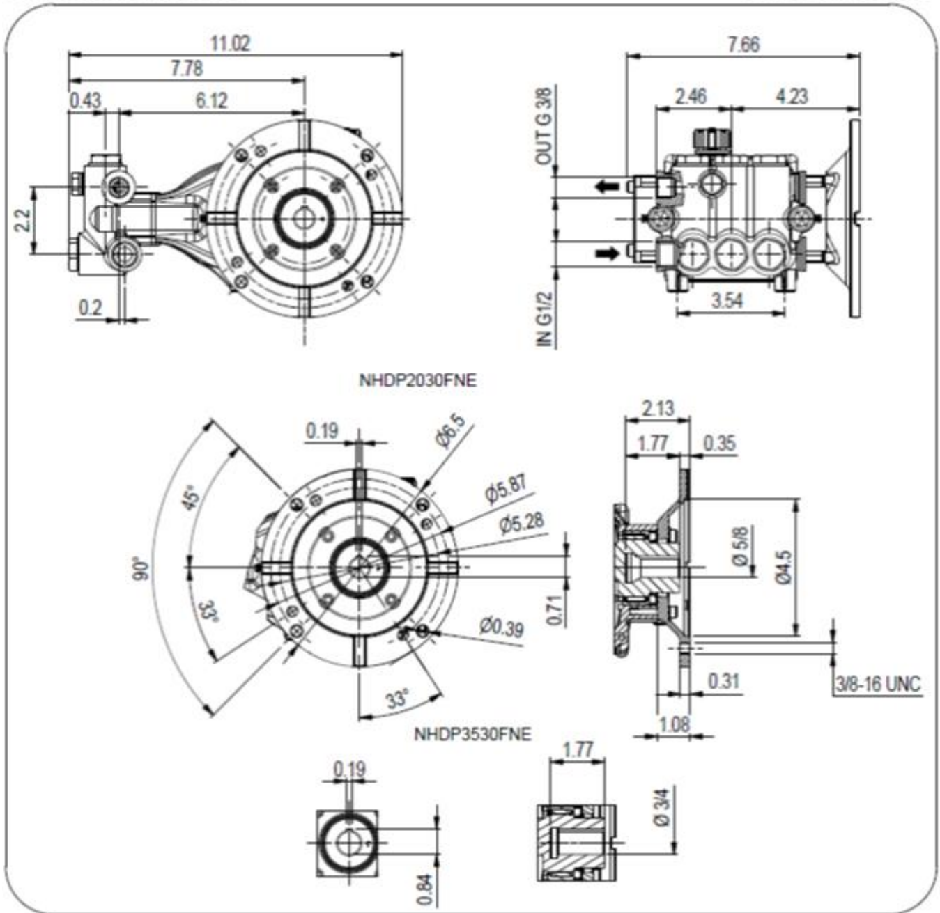
Dimensioni d'ingombro
